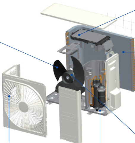
Serration fan
